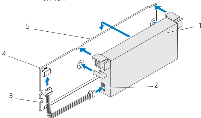
図 3-5. TBBU の取り付け
