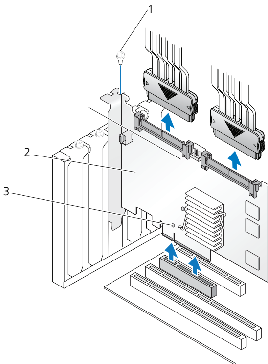
図 3-8. PERC 6/i アダプタの取り外し
