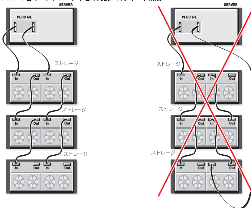
図 3-13. 3 台のエンクロージャとの冗長パスサポート構成
