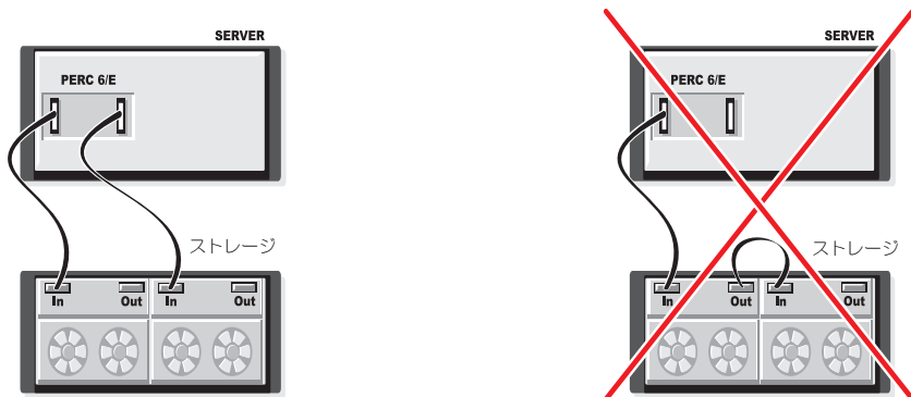
図 3-11. 1 台のエンクローチャとの冗長パスサポート構成
