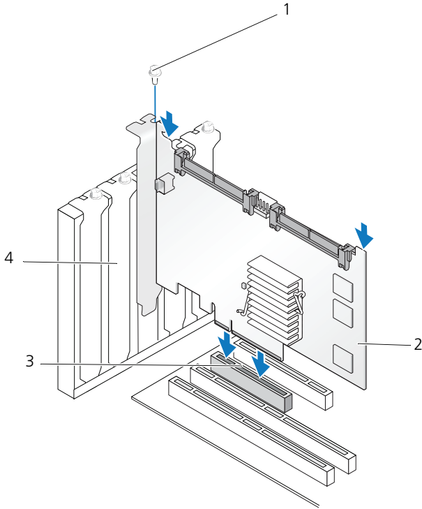
図 3-2. PERC 6/i アダプタの取り付け
