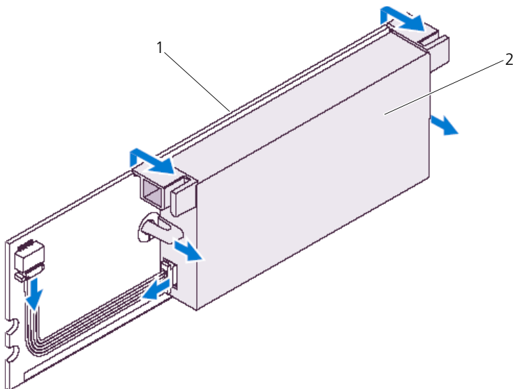
図 3-10. TBBU の取り外し
