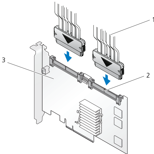
図 3-4. コントローラへのケーブルの接続
