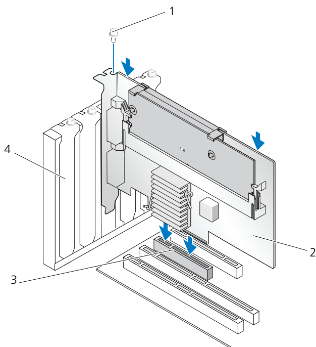
図 3-1. PERC 6/E アダプタの取り付け
