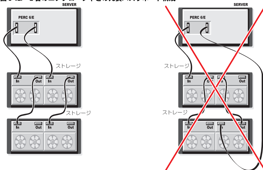
図 3-12. 2 台のエンクローチャとの冗長パスサポート構成
