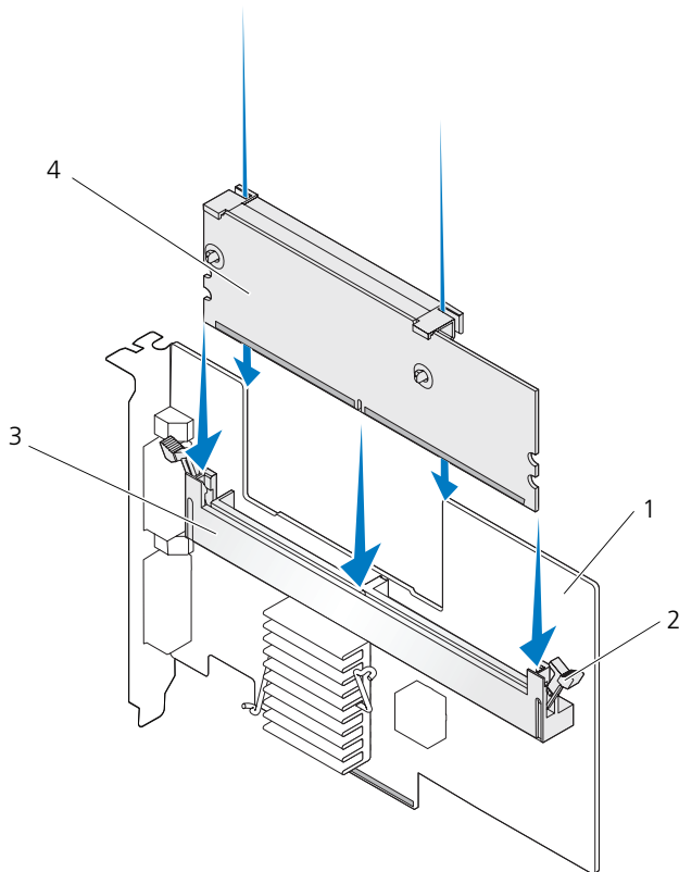
図 3-6. DIMM の取り付け
