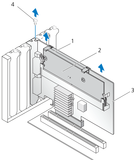
図 3-7. PERC 6/E アダプタの取り外し
