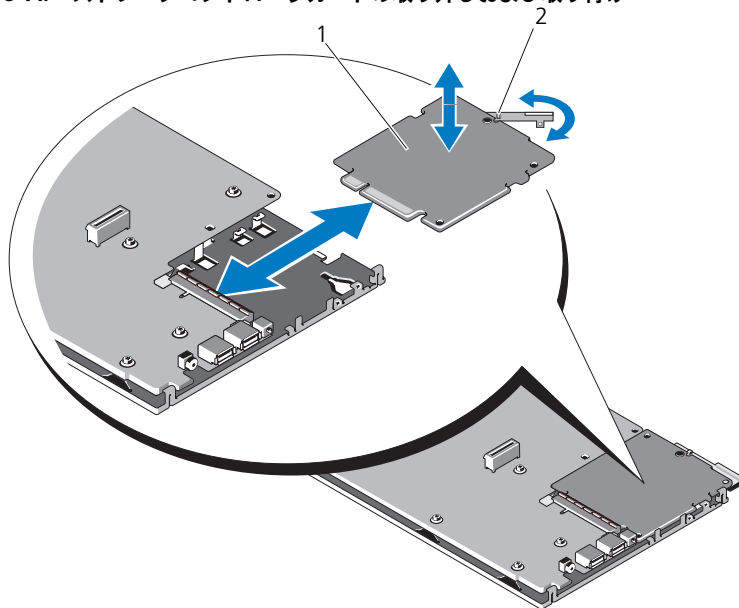
図 3-14. ストレージコントローラカードの取り外しおよび取り付け
