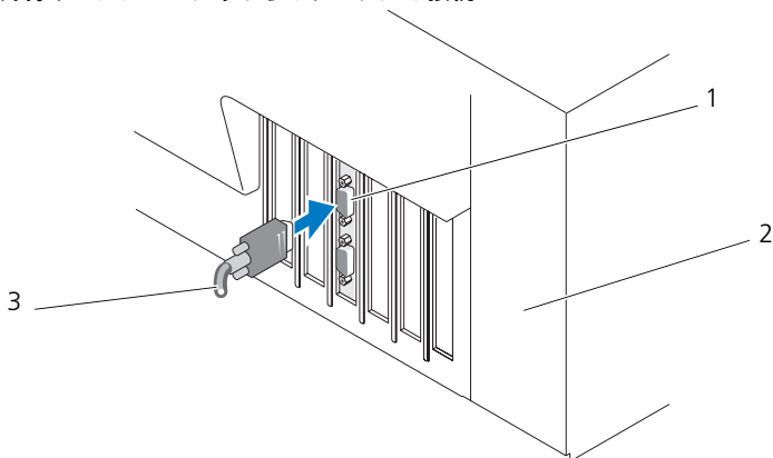
図 3-3. 外付けエンクロージャからのケーブルの接続
